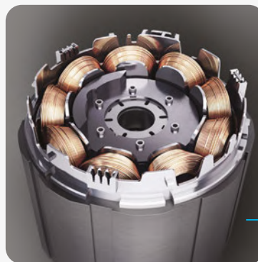
BLDC роторен
